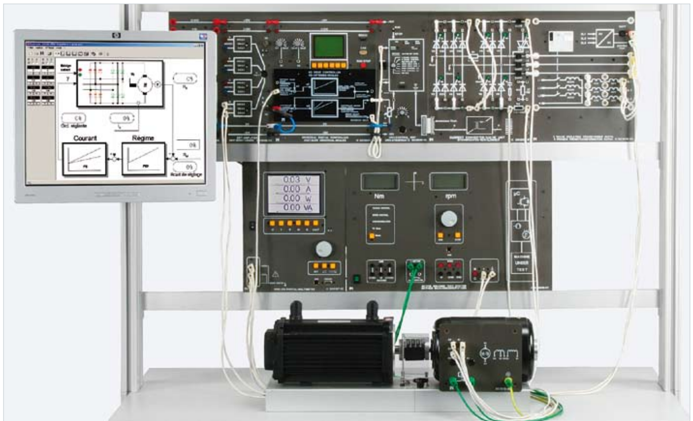
Exemple d'expérience « Régulation de la vitesse de rotation d'un moteur à courant continu EPE 11 »
