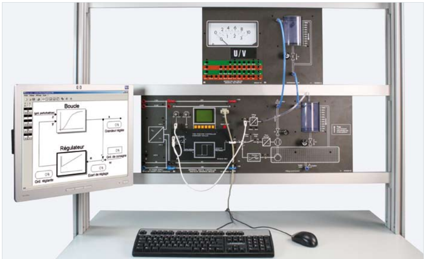
Exemple d'expérience « Régulation de niveau IAC 10 »
