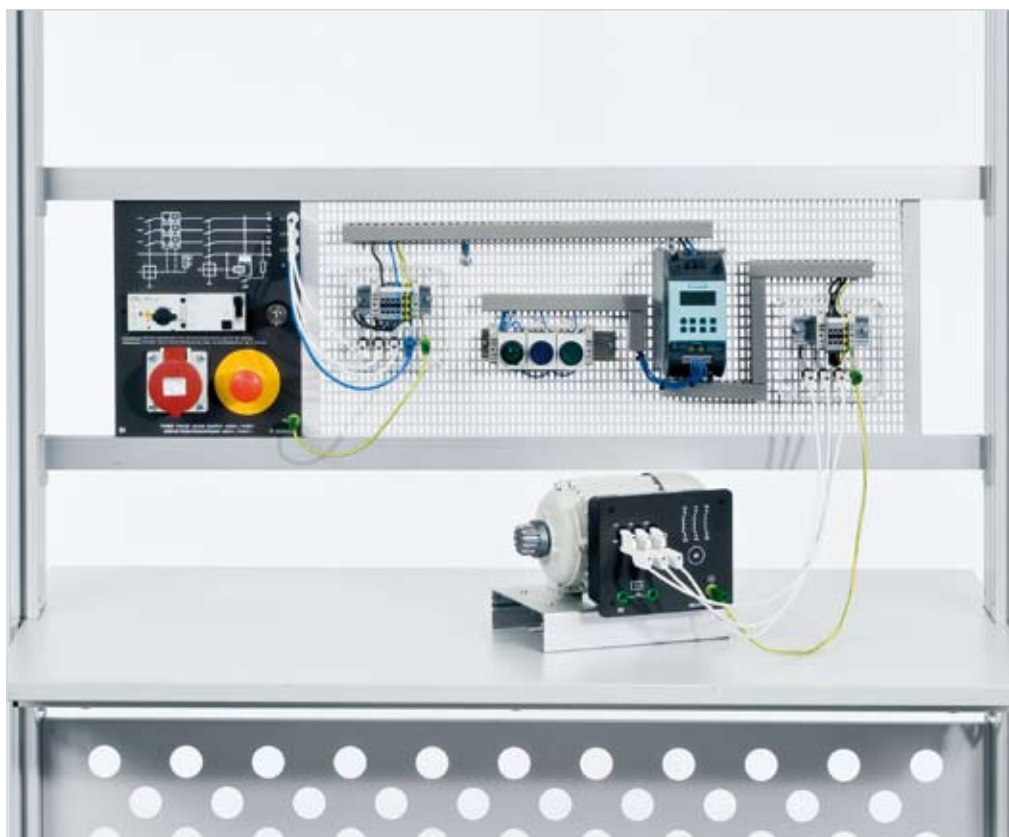
Système d'exercices de montage
